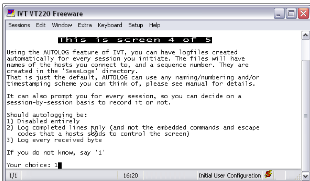
Рисунок 3.11: Шаг 4 – выбор режима регистрации сессий (функция AUTOLOG)
