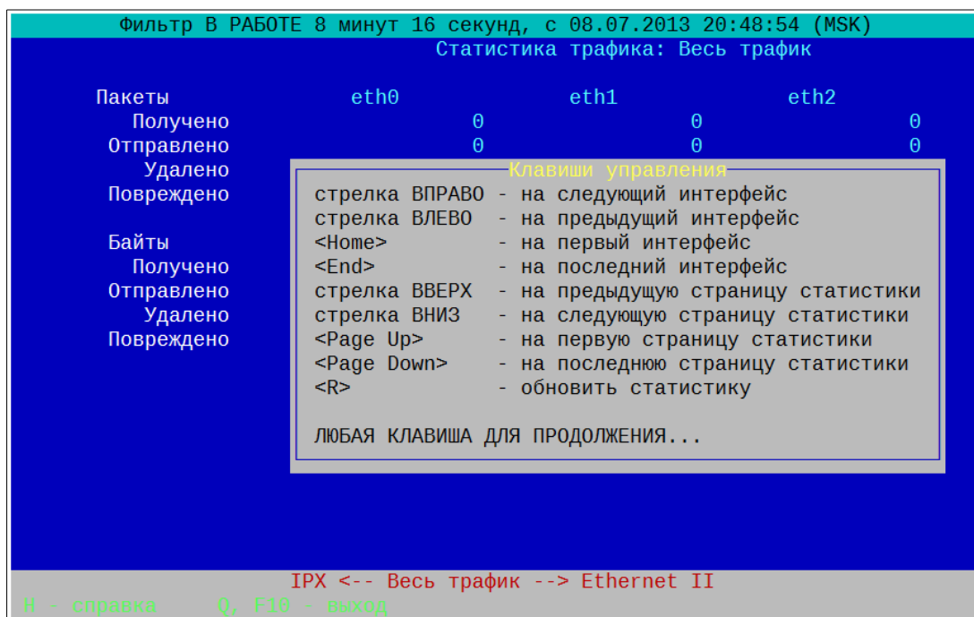
Рисунок 3.45: Состояние пакетного фильтра и статистика трафика
