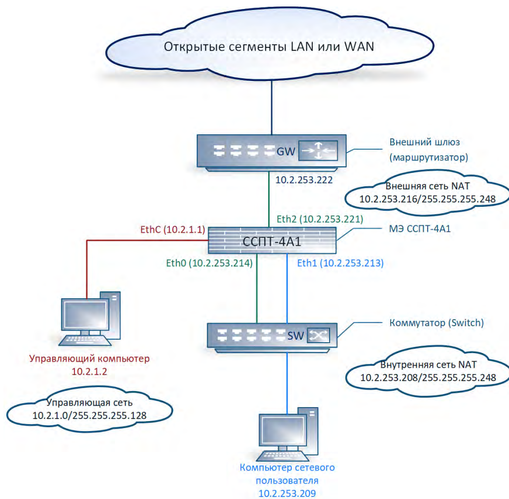
Рисунок 3.15: HTTP-посредник. Схема подключения с использованием NAT
