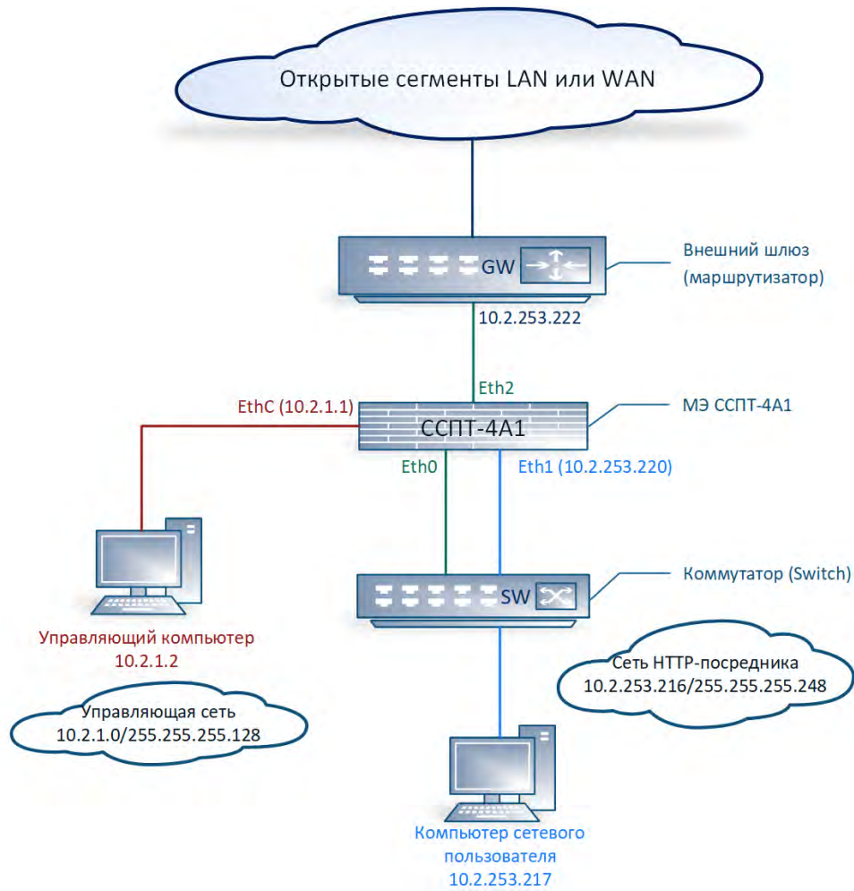
Рисунок 3.14: HTTP-посредник. Схема подключения без использования NAT
